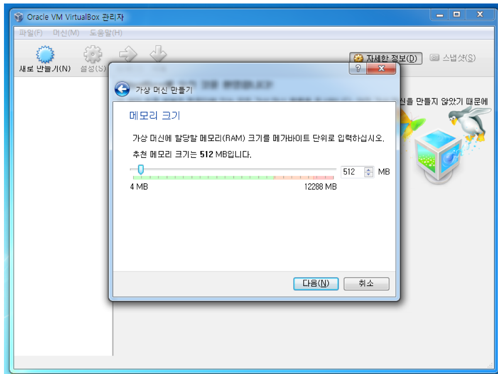
사진 12: 메모리 설정
