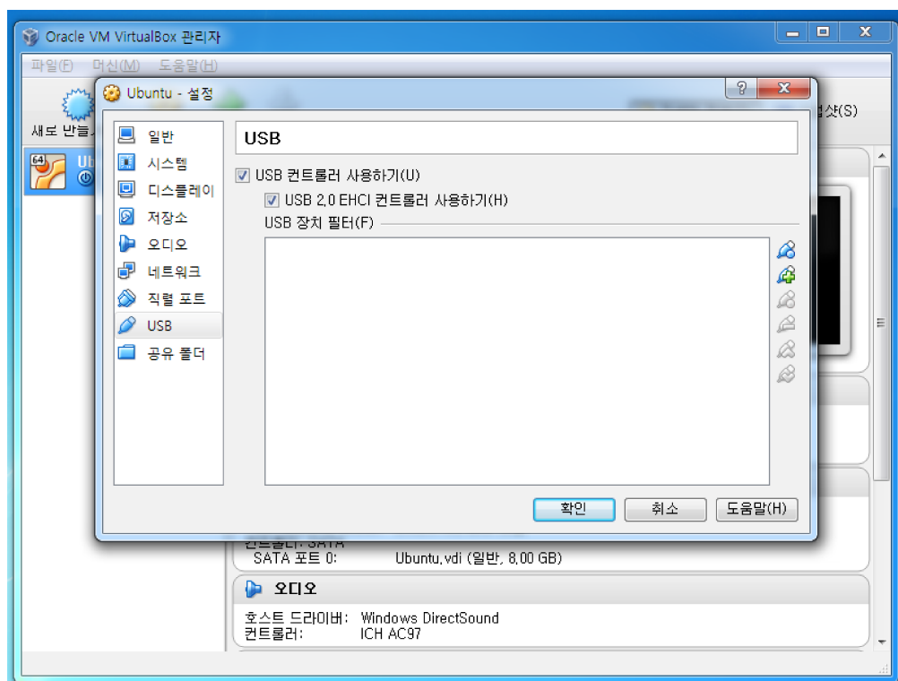
사진 28: 이상 없음!
