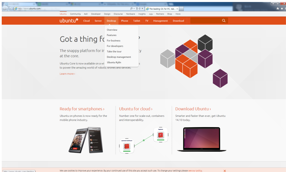
사진 15: Ubuntu Desktop
