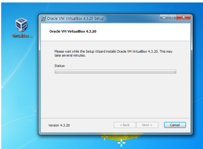
사진 7: VirtualBox 설치중
