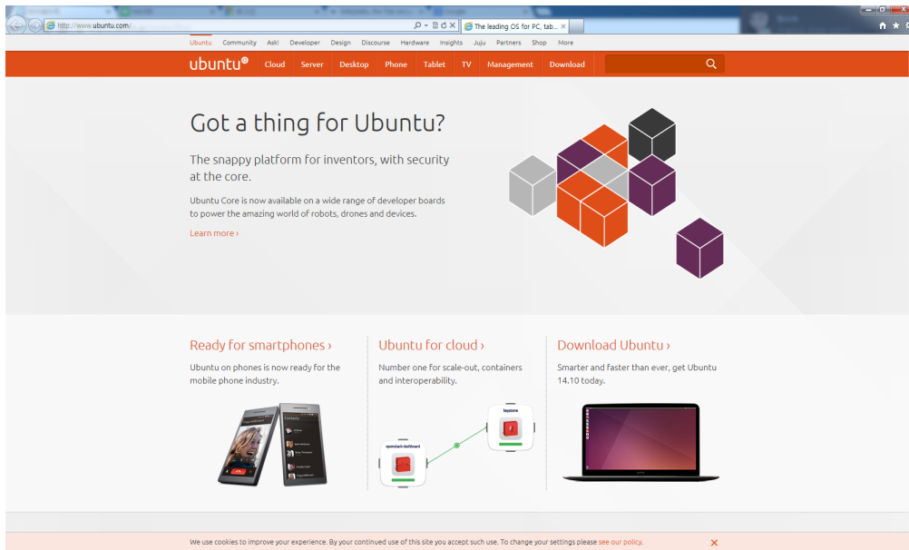
사진 14: http://www.ubuntu.com
