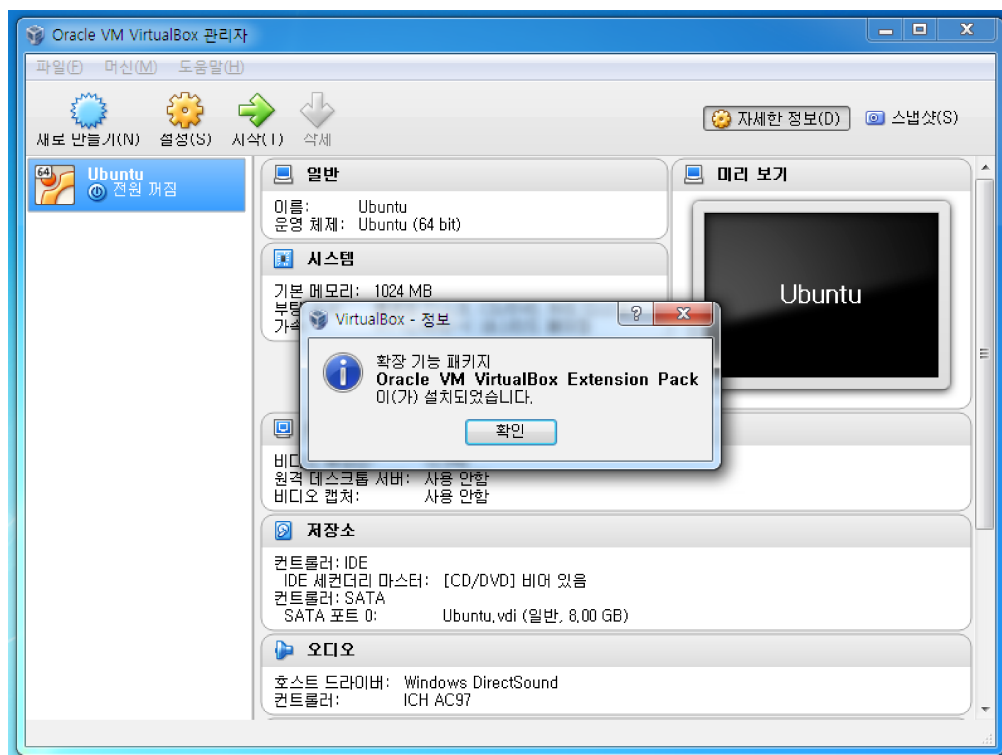
사진 27: 설치 끝
