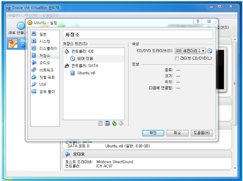
사진 19: 가상머신 설정화면
