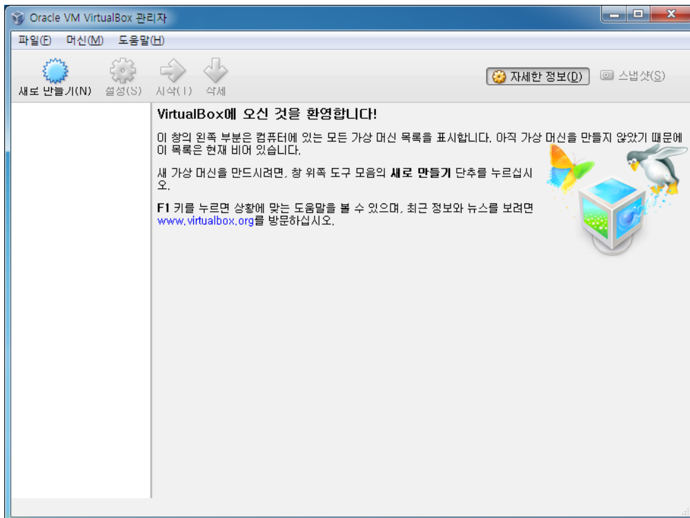
사진 10: VirtualBox
