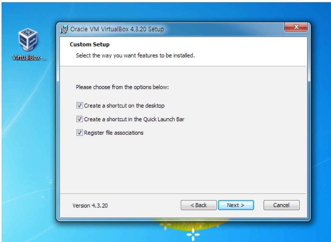
사진 5: 바로가기 생성
