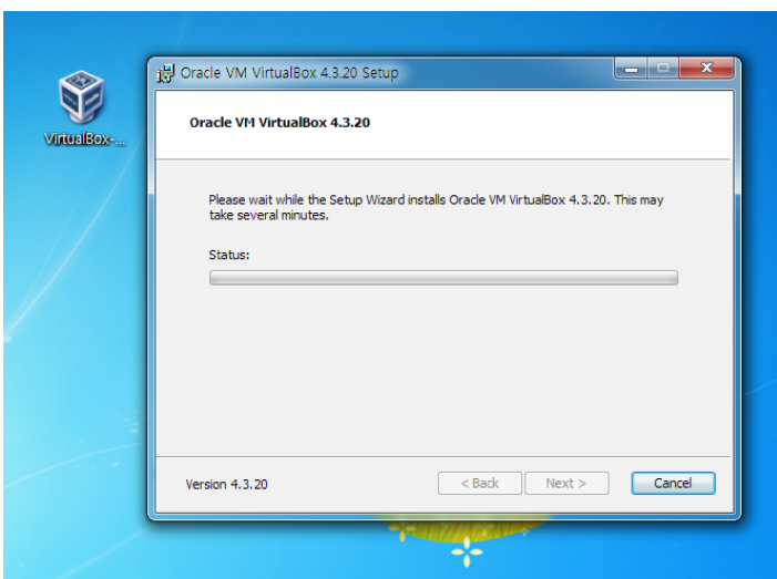
사진 7: VirtualBox 설치중
